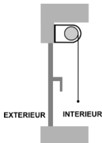
Tissu éloigné de la vitre (Enroulement extérieur)
