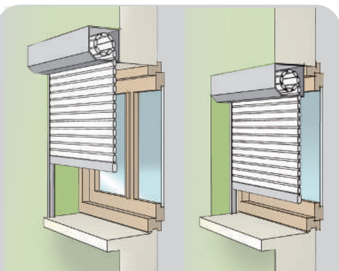
Pose en façade
