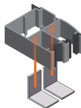
arrêt bas de coulisse (arrête le tablier ou le store lorsque que la coulisse est en pose façade)
