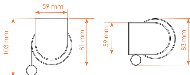
barre de charge occulte (ronde)
