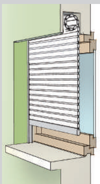
Enroulement extérieur
