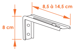
équerre murale courte (8,5 à 14,5 cm)
