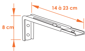
équerre murale longue (14 à 23 cm)
