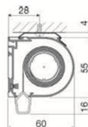
Pose plafond
