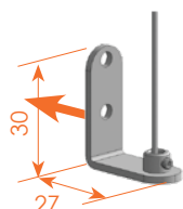
pose de face ou en tableau
