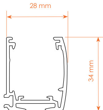
Profil haut pour la manœuvre chaînette
