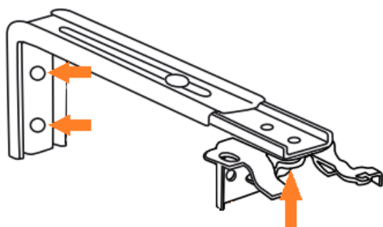
Fixation de face avec équerres de 6 à 9,5 cm ou 8,5 à 14,5 cm ou de 14 à 23 cm
