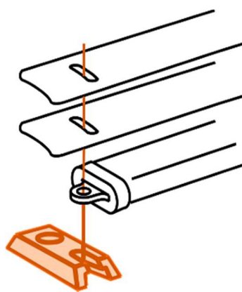
Guidage câbles avec pontets (au sol)
