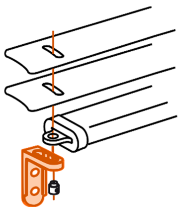
Guidage câbles avec équerres
