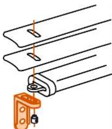
Guidage câbles avec équerres
