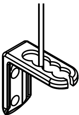
Guidage par câbles avec équerres
